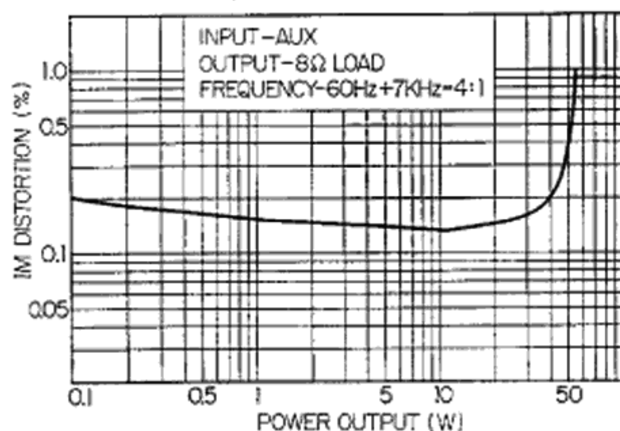
IM DISTORTION
